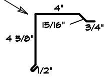
4b 2X4 MINI GABLE
